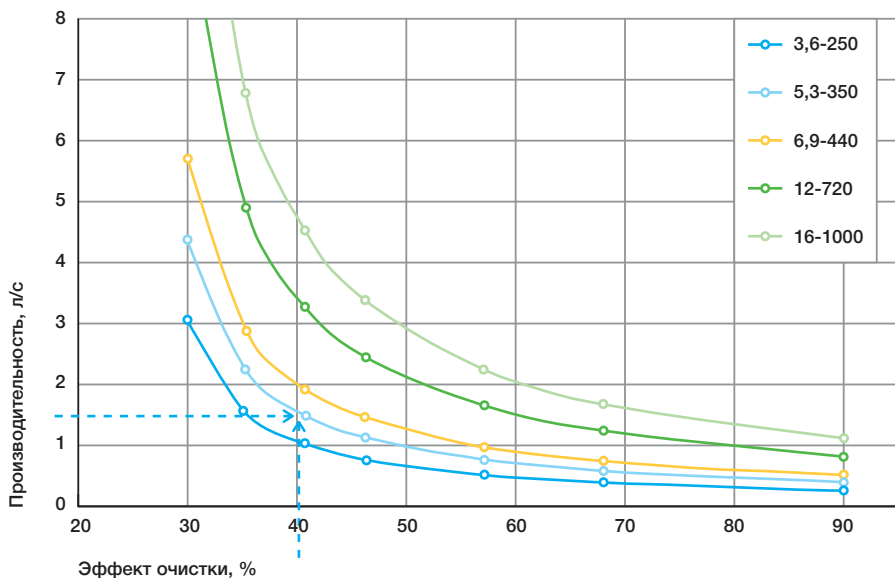
Диаграмма производительности жиросовкателей Евролос Норма
